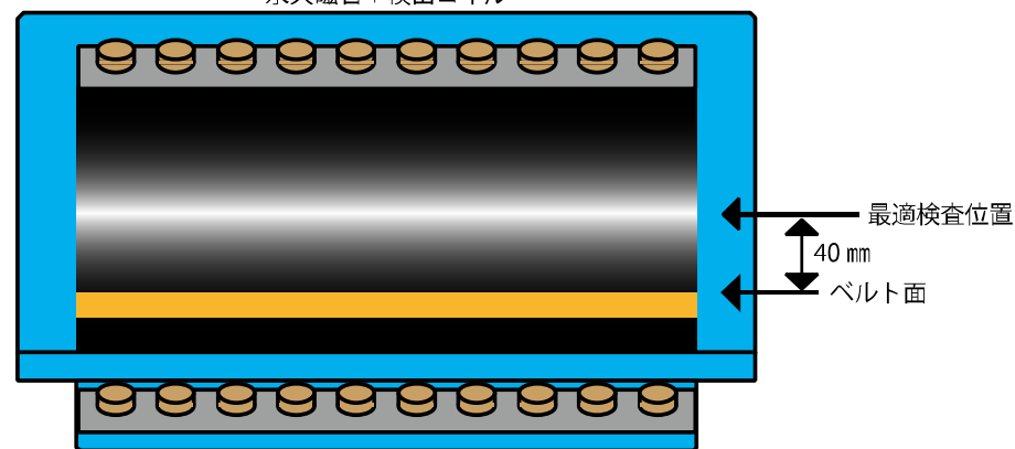
永久磁石+検出コイル
