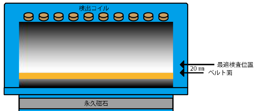
センサーヘッド断面図
