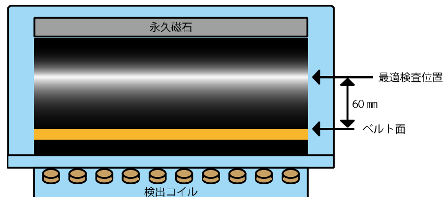
センサーヘッド断面図
